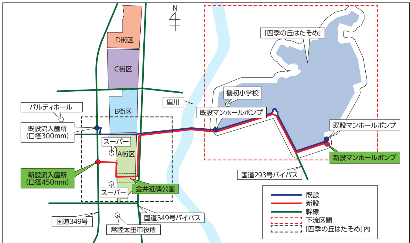
公共下水道事業(四季の丘はたそめ区域)改修ルート図
