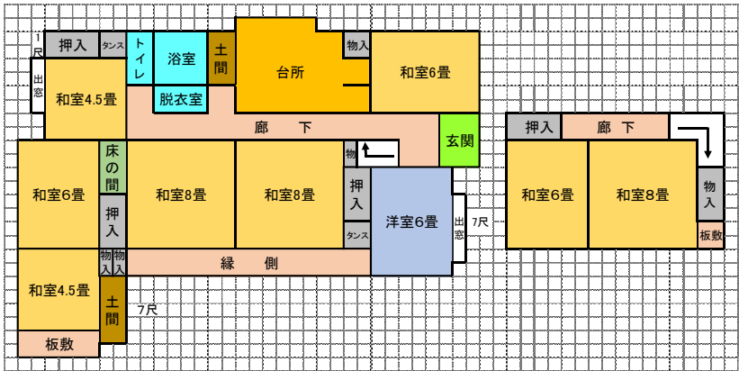
1階
