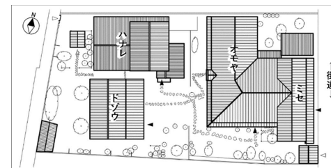
配置図
