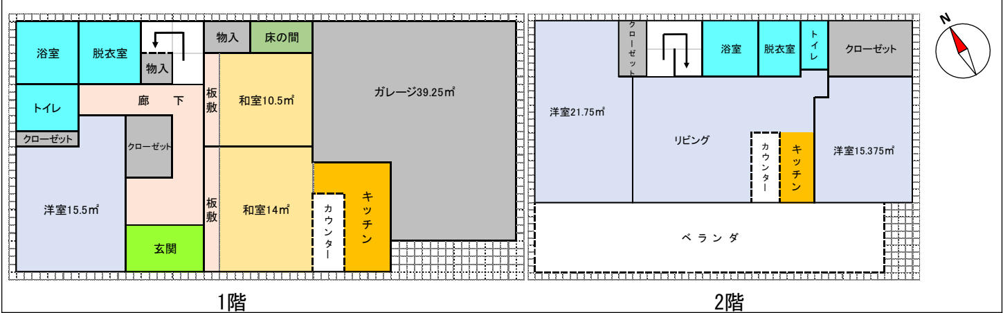
1階 2階
