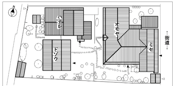
配置図
